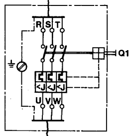
WIRING DIAGRAM FOR SCHALTPLAN FÜR 80800 KGE
