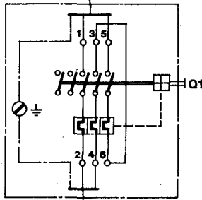
WIRING DIAGRAM FOR SCHALTPLAN FÜR 80800 KA AND/UND KT
